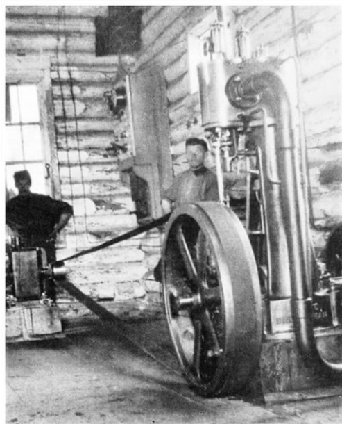
Электростанция на Варваинском промысле А.Г. Гансберга
