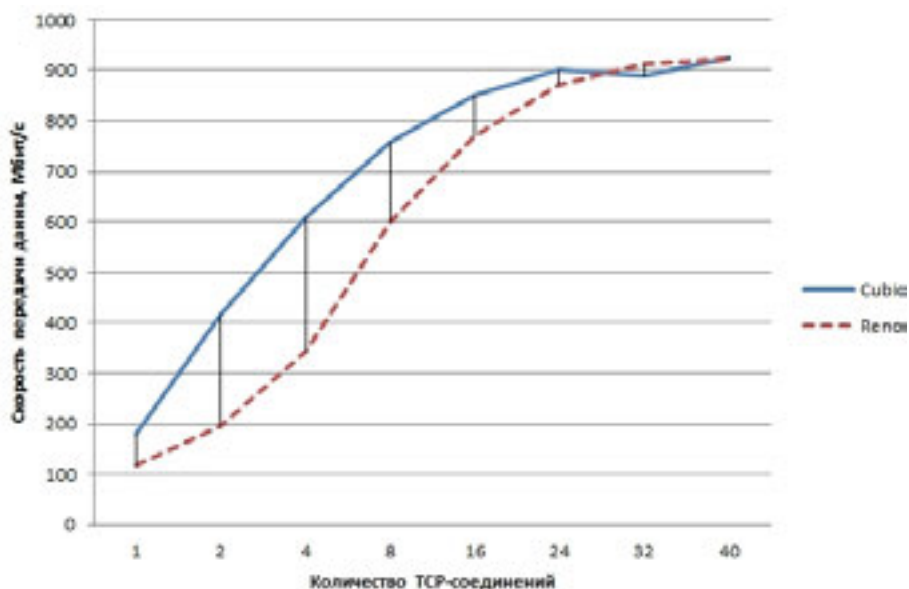
Рис. 6. Зависимость скорости передачи данных от количества соединений
