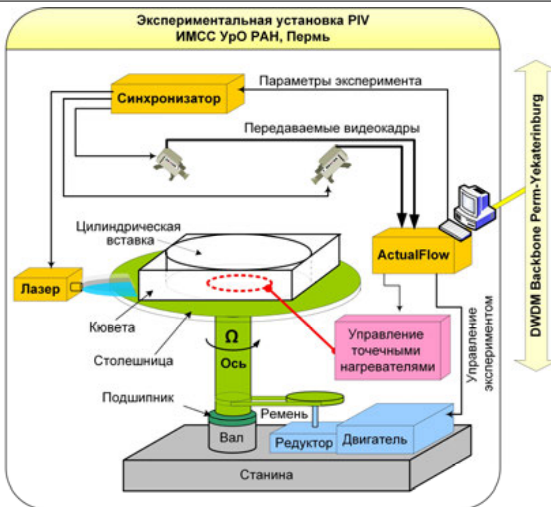
Рис. 14. PIV-экспериментальная установка
