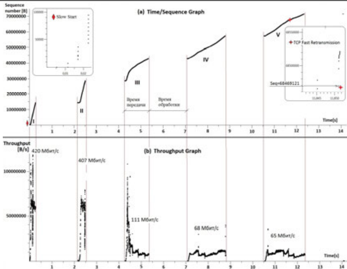
Рис. 5. Wireshark, импульсный трафик (Sequence number – порядковый номер байта в потоке)
