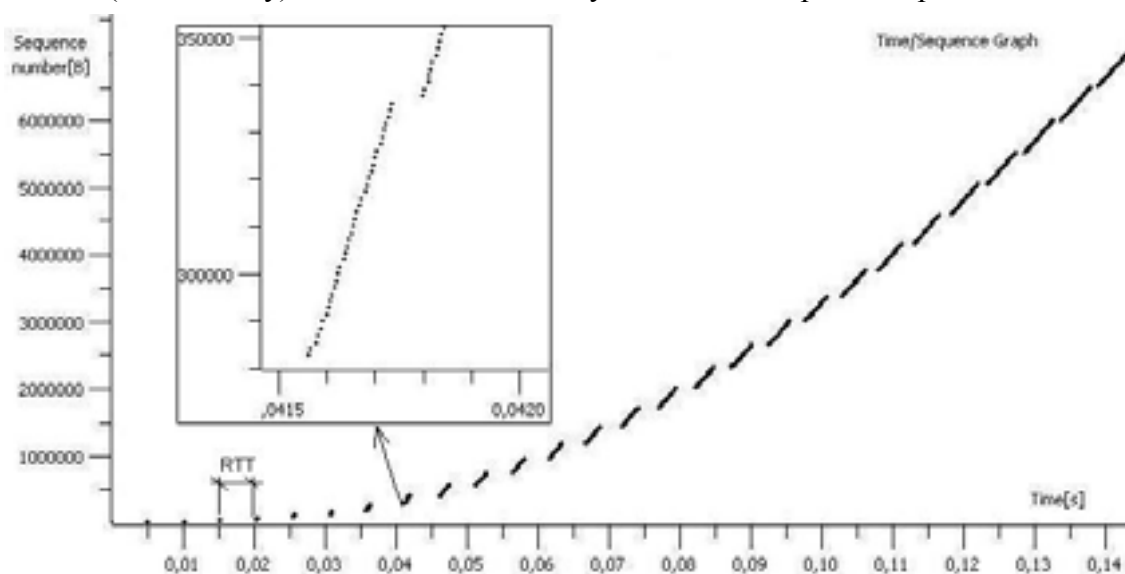
Рис. 4. Медленный старт TCP, RTT = 5 мс, скорость канала 1 Гбит/с
