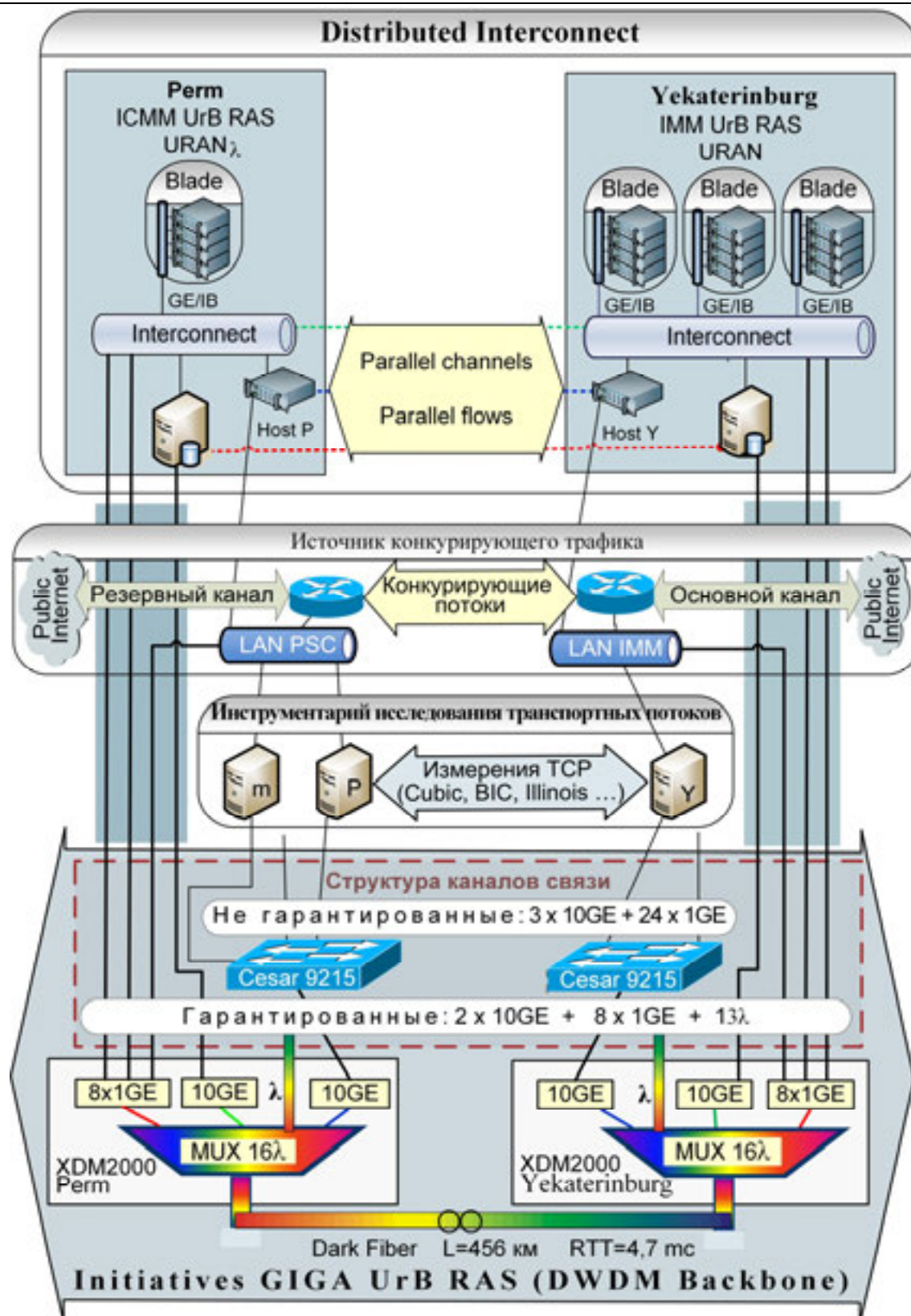
Рис. 3. Структура каналов связи
