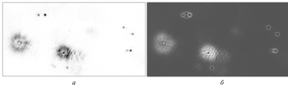
Рис. 16. Применение вейвлет-обработки для анализа изображений: а – исходное изображение; б – результат обработки (распределение вейвлет-коэффициентов). Окружности показывают пары бликов, по которым производится восстановление размеров капель
