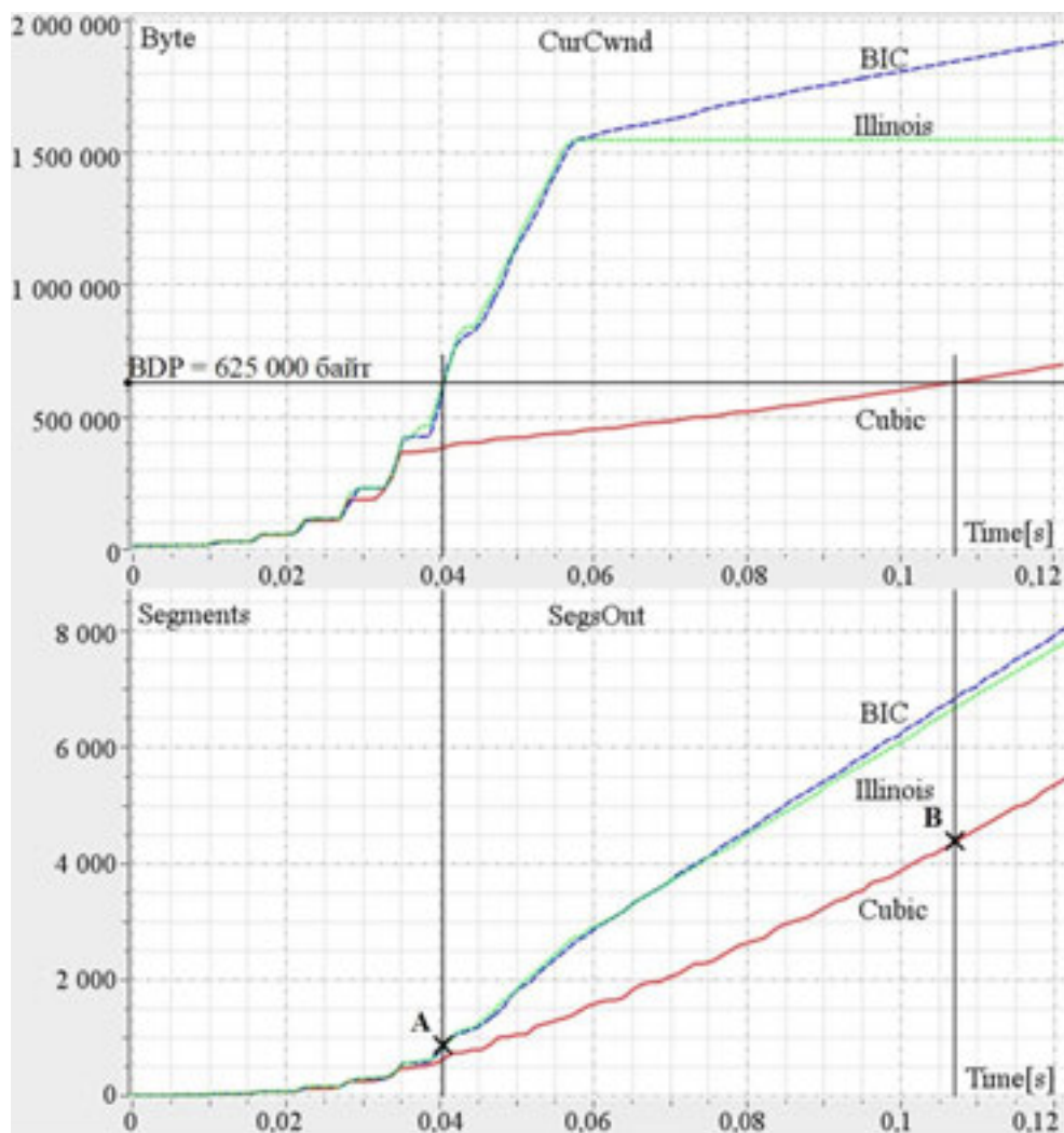
Рис. 8. Сравнение динамики изменения параметров TCP в области медленного старта
