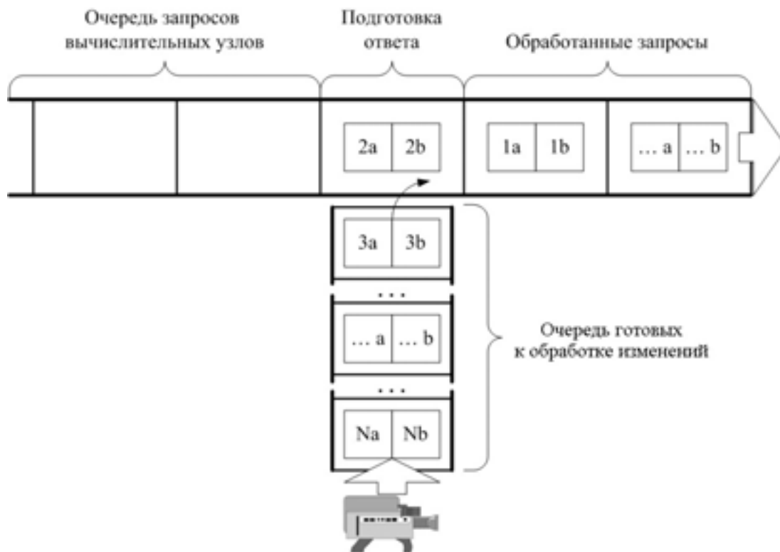
Рис. 10. Распределение данных в ответ на запросы вычислительных узлов
