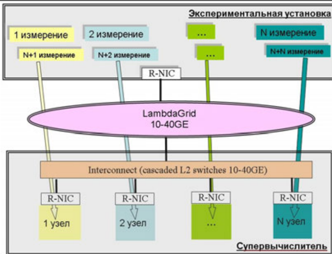
Рис. 9. Идеальная модель обработки структурированного потока данных
