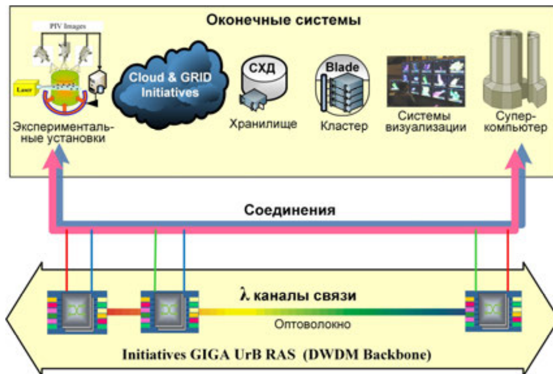
Рис. 1. Территориальная киберинфраструктура Урала
