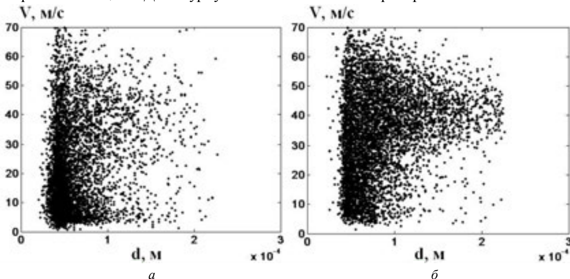
Рис. 19. Распределение капель в плоскости V - d : а – для p = 0,1 атм., б – для p = 10 атм.
