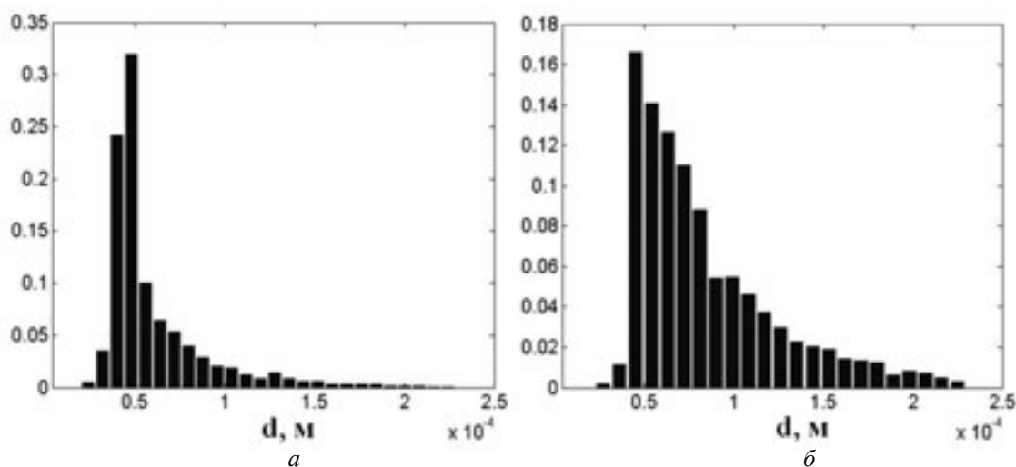
Рис. 18. Распределение капель по размерам, а – для p = 0,1 \text{ атм.} , б – для p = 10 \text{ атм.} , по вертикали отложена относительная доля капель
