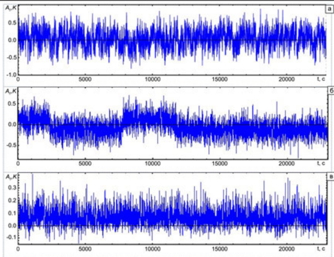
Рис. 20. Вариации амплитуды крупномасштабных пульсаций температуры при Ra = 4,4 \cdot 10^9 в полостях с различной геометрией: \Gamma = 0,1 (смешанный режим) (а), \Gamma = 0,2 (режим с инверсиями) (б), \Gamma = 1,0 (режим без инверсий) (в)
