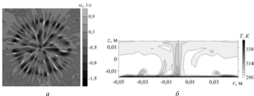
Рис. 15. Поле радиальной компоненты завихренности на высоте h = 3 мм (а), всплывающие конвективные струи в центральном вертикальном сечении (б)
