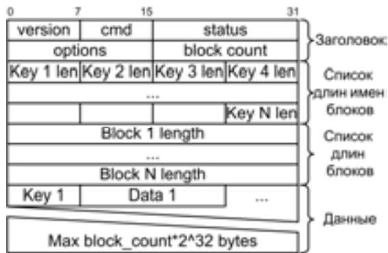
Рис. 11. Формат пакета протокола SciMP
